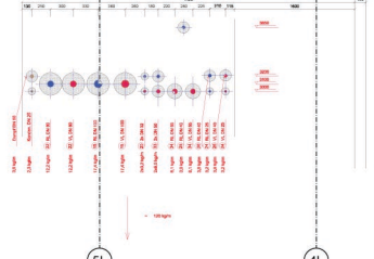
SCHNITT C-C M 1:20
